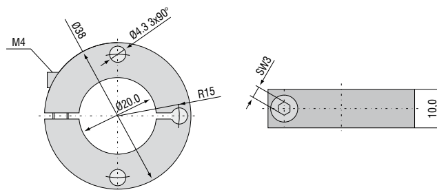
Flange DTA-F20
